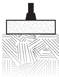
Betoonvundament
